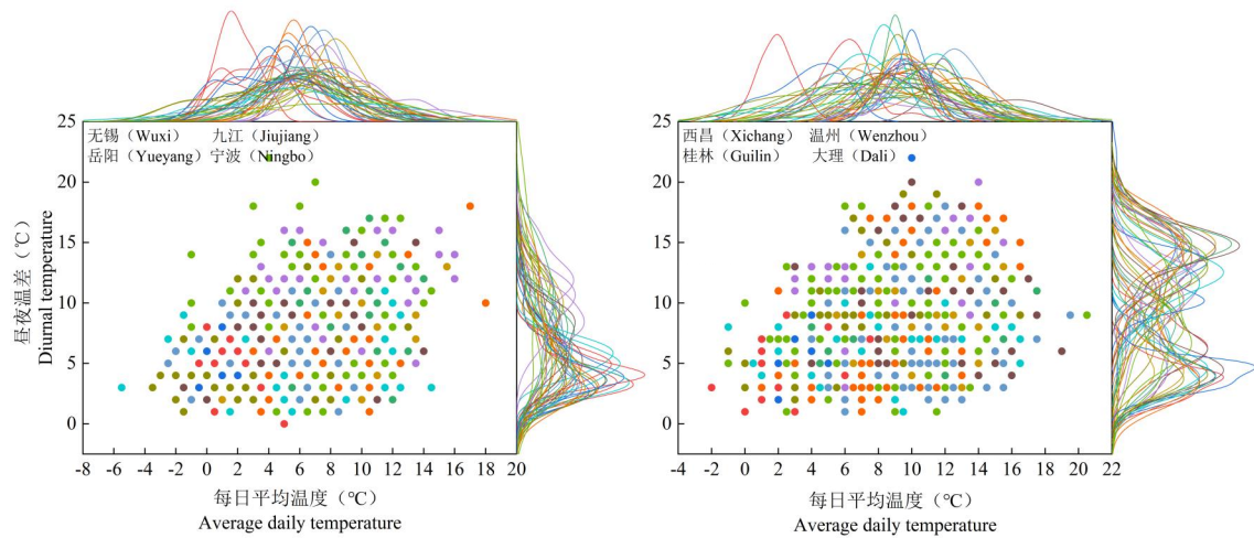
图 1 2011-2021 年 1 月平均气温为 10、6℃下地区昼夜温差（数据来源于 www.tianqi.com）
