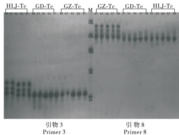
图 4 退火温度对螟黄赤眼蜂 3 个地理种群微卫星鉴定结果的影响
