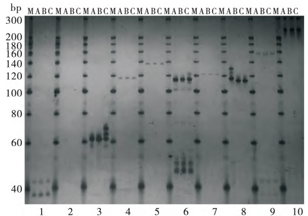
图 2 螟黄赤眼蜂 3 个地理种群的引物筛选结果
