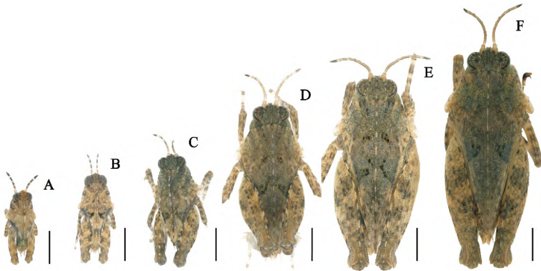
图 2 日本蚱的雄性若虫及成虫
