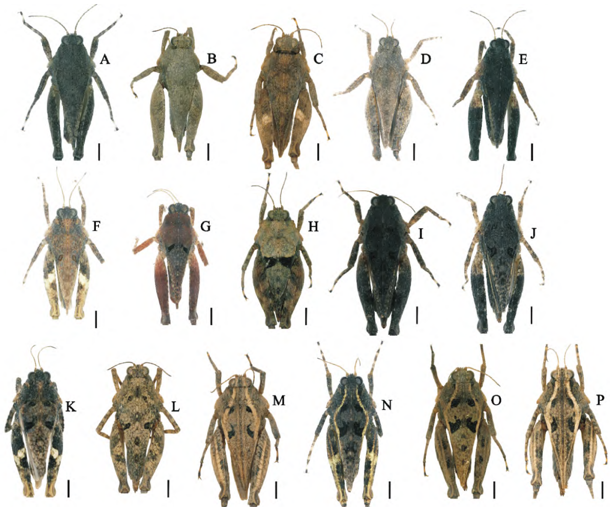
图 5 日本蚱前胸背板斑纹的多态性
