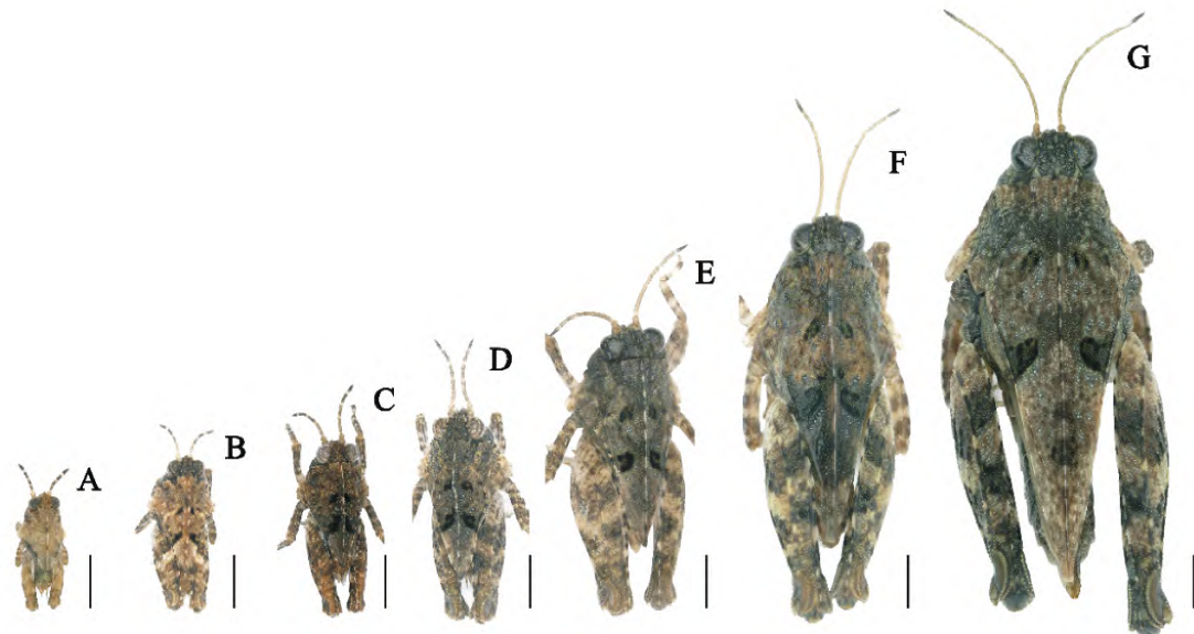
图3 日本蚱雌性若虫及成虫
