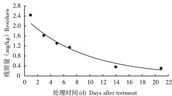
图 2 噻虫嗪的最终残留动态
